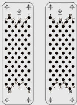
接插针排序
